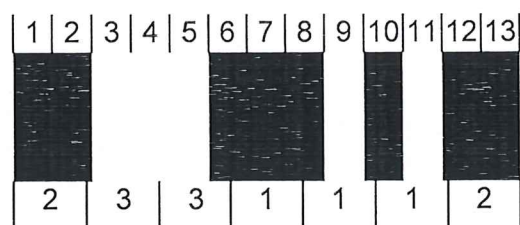
Hình 13 – Ký tự vạch xác định dạng của mã vạch 128
