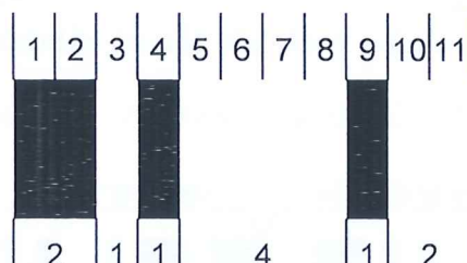
Hình 11 – Ký tự xác định bắt đầu A của mã vạch 128
