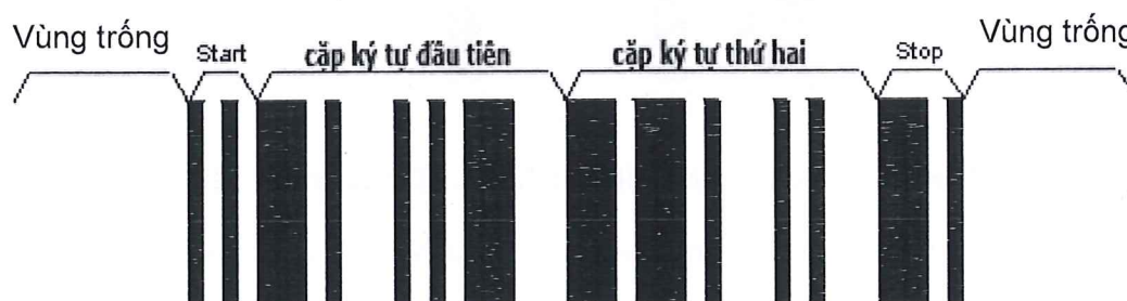
Hình 9 – Mã vạch ITF gồm cả các vùng trống.
